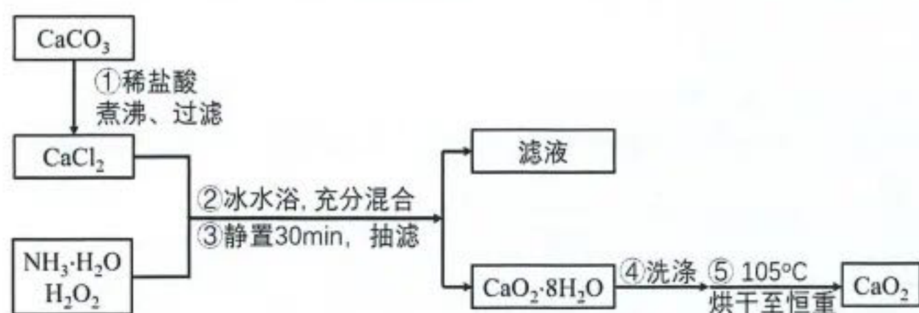
图 2.1 过氧化钙制备流程图
