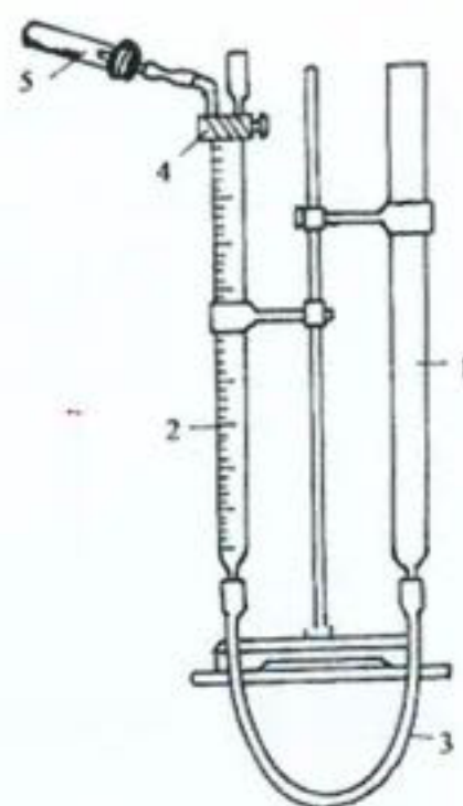
图 2.2 量气法装置图
