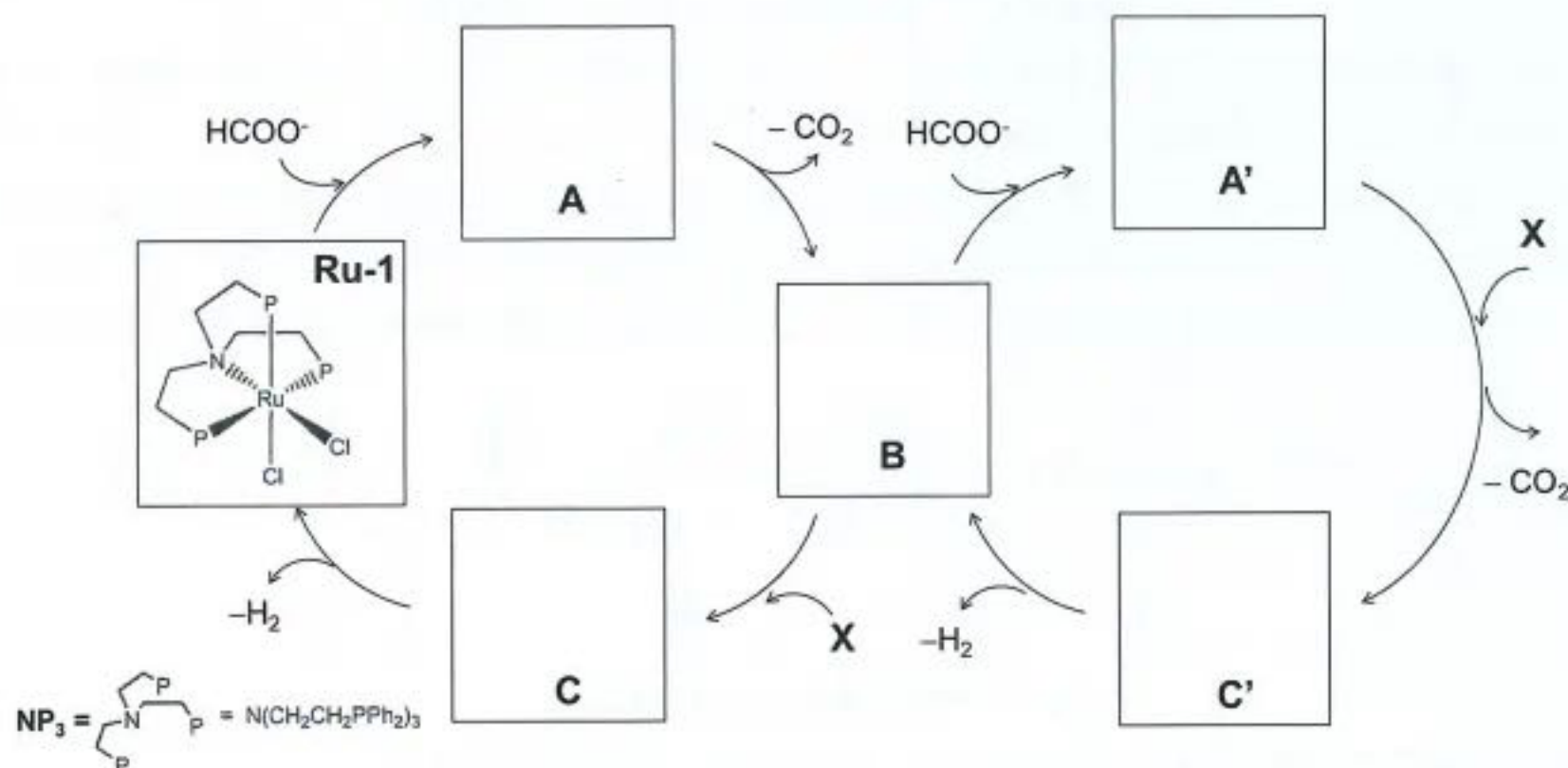
图 3.2 过渡金属催化的甲酸脱羧反应
