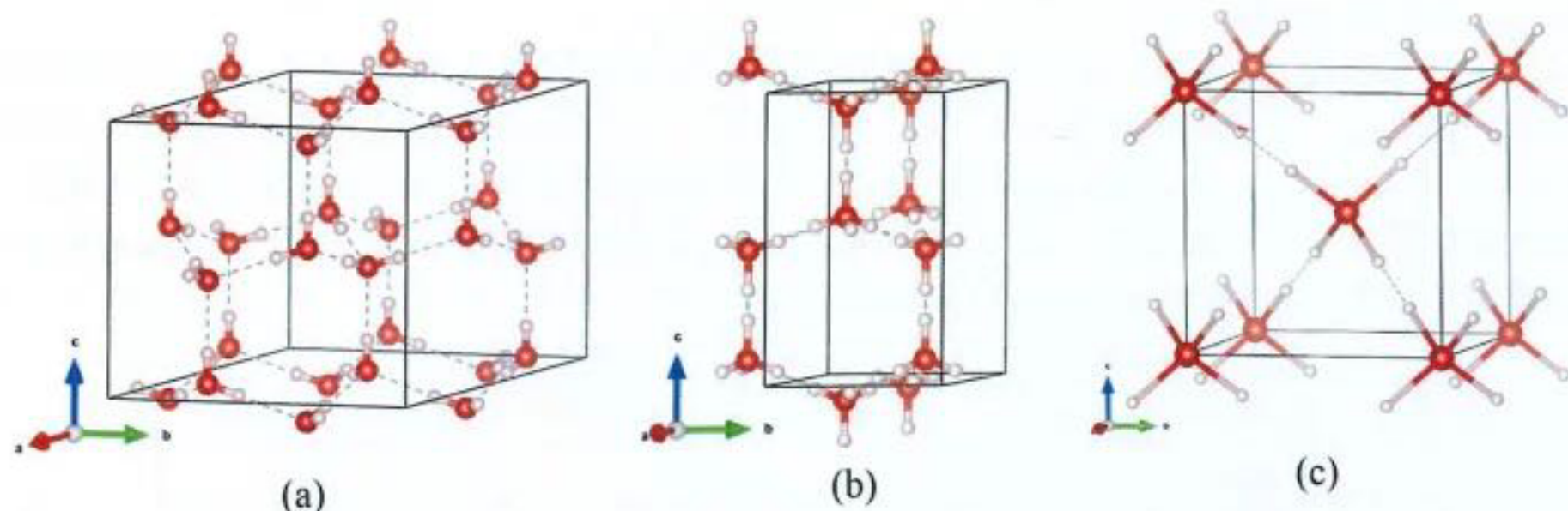
图 5.1 几种冰的结构
