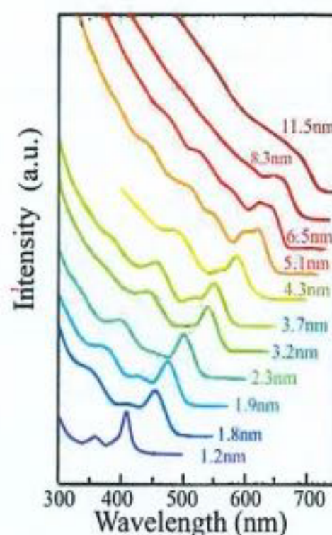
图 6.1 CdSe 的吸收光谱
