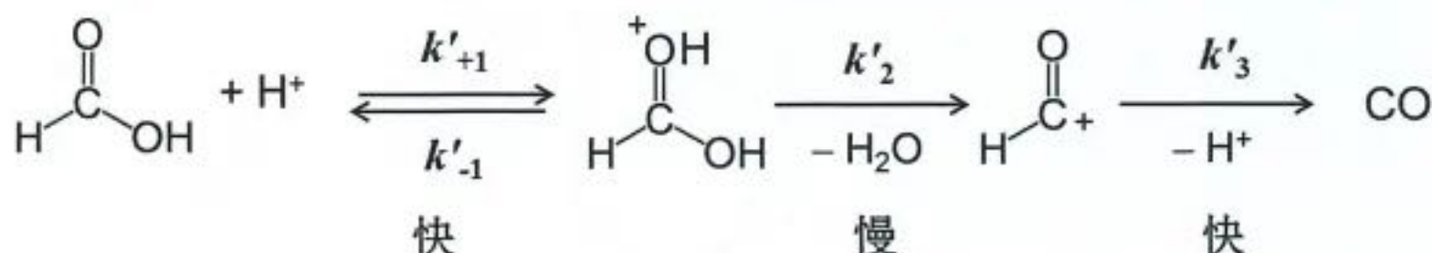
图 3.1 甲酸水热脱水反应的机理
